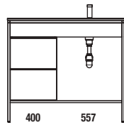
LAVABO COQUETA A LA IZQUIERDA
