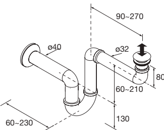
LAVABO POZA CENTRADA (1 o 2 coquetas)
